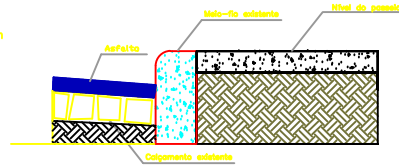
Detalhe do meio fio, trecho com calçamento
