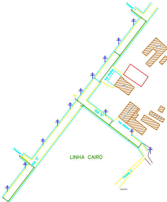
PLANTA BAIXA ESCALA: 1:1.000
